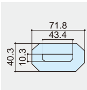
Dimensions
